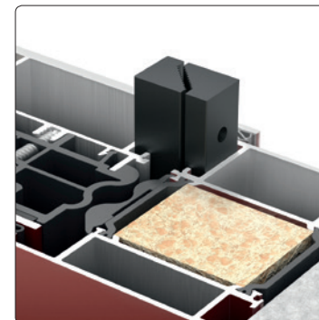
5-fache Keilsperrrensicherung an der Bandseite
